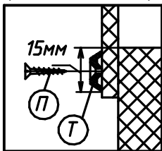
Крепление задней стенки к детали №324 (комплект №10)
