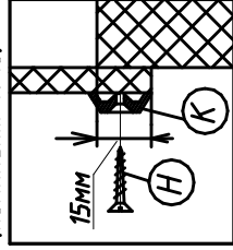
Крепление задней стенки к №611,610 (комплект №10)
