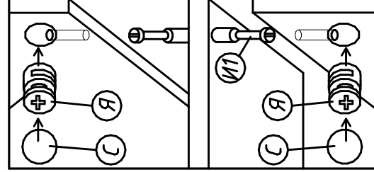
Крепление стяжки эксцентриковой (комплект №45А)
