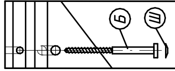
Крепление винта саморезного (комплект №19)
