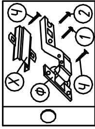
Крепление петли (комплект №4)
