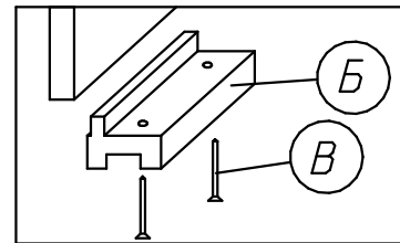
Крепление стяжки эксцентриковой (комплект №45)
