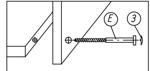
Крепление винта саморезного (комплект №19)
