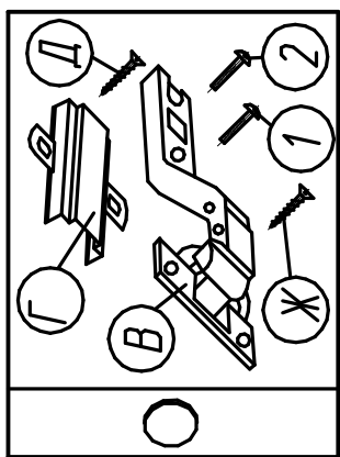
Крепление петель (комплект №4)
