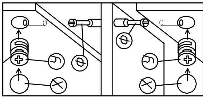
Крепление стяжки эксцентриквой (комплект №45)
