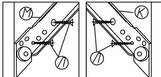
Крепление роликовой направляющей левая (комплект №25) правая
