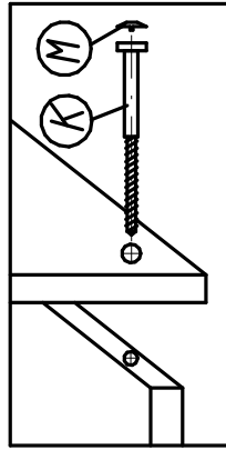
Крепление винта саморезного (комплект №19)
