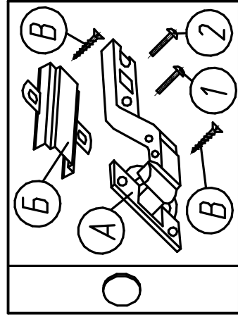
Крепление петли (комплект №4)
