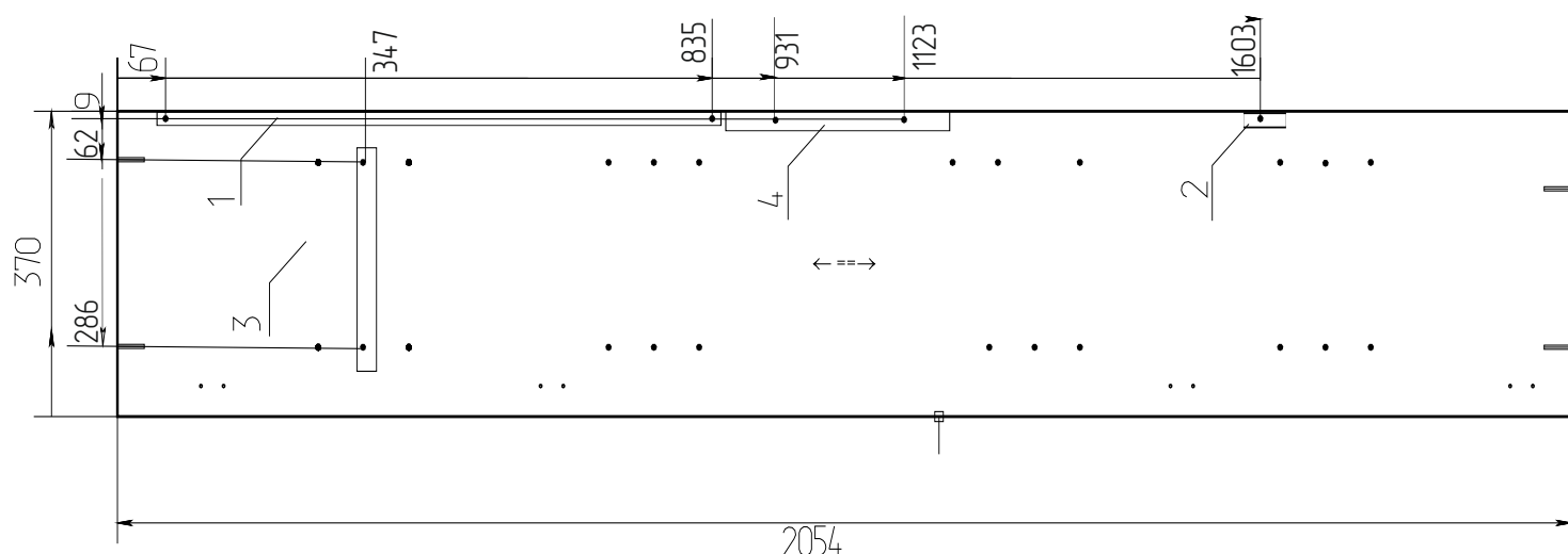
Деталь №1
